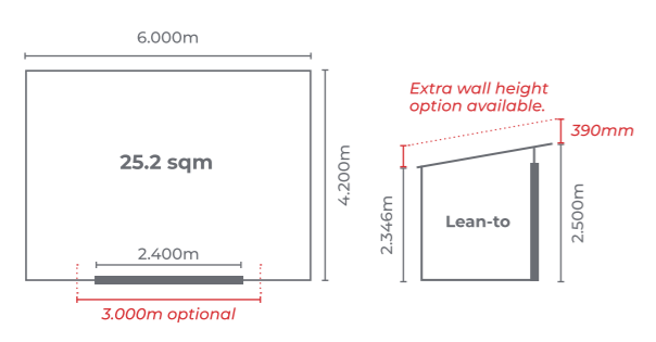
Kapiti 6m x 4.2m DLL6042 Kapiti Extra Height DLLEH6042
